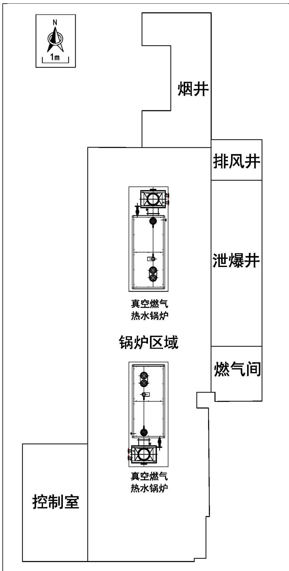
附图 4 锅炉房平面布置图
