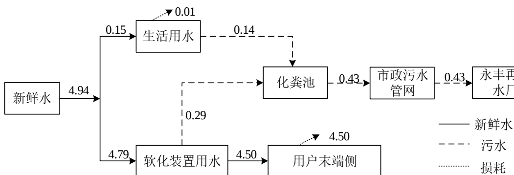
图 2-2 本项目日水平衡图 (m³/d)
