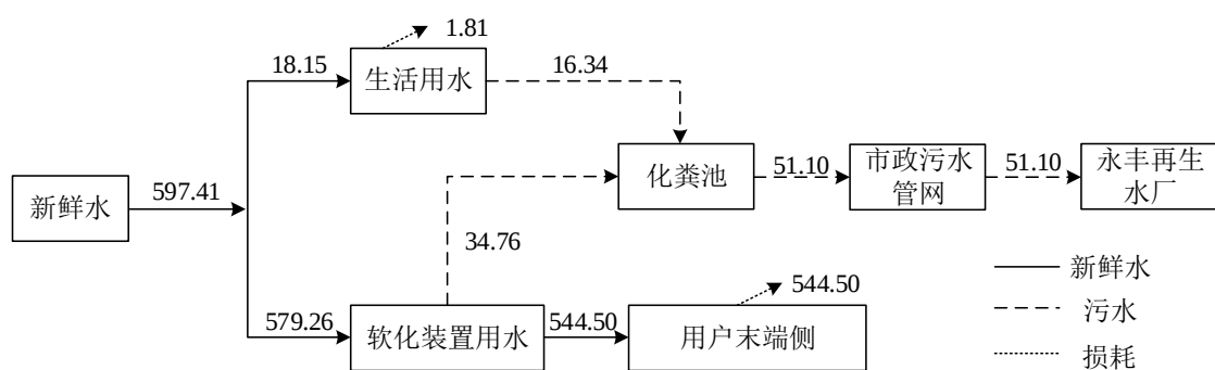
图 2-1 本项目年水平衡图 (m³/a)
