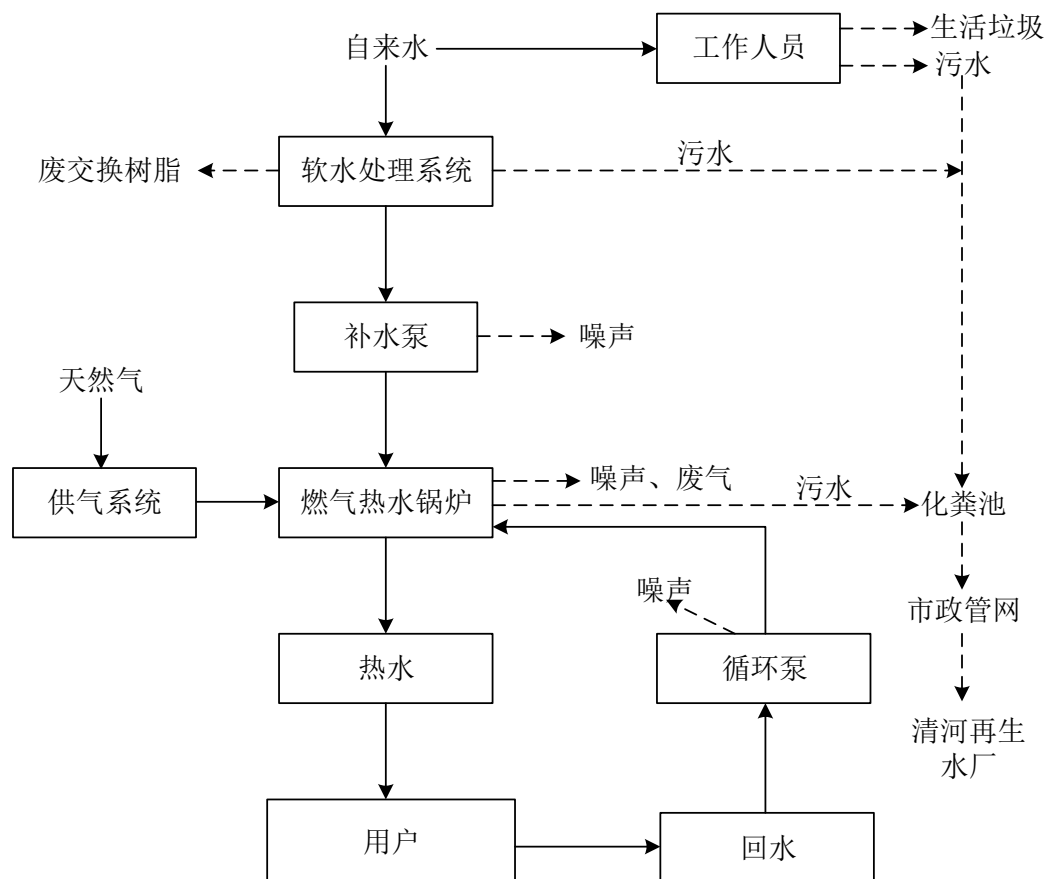
图 2-4 项目工艺流程及产污环节图
